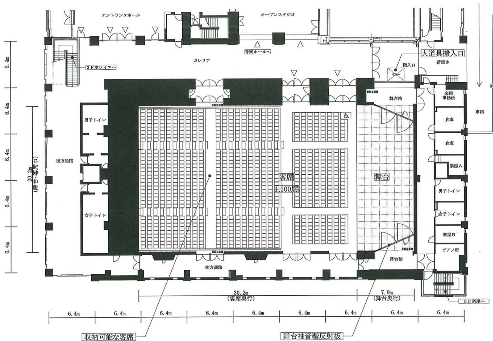
2階平面図
